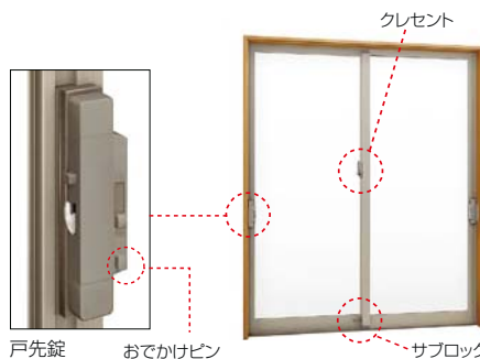
戸先錠
