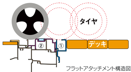
フラットアタッチメント構造図
